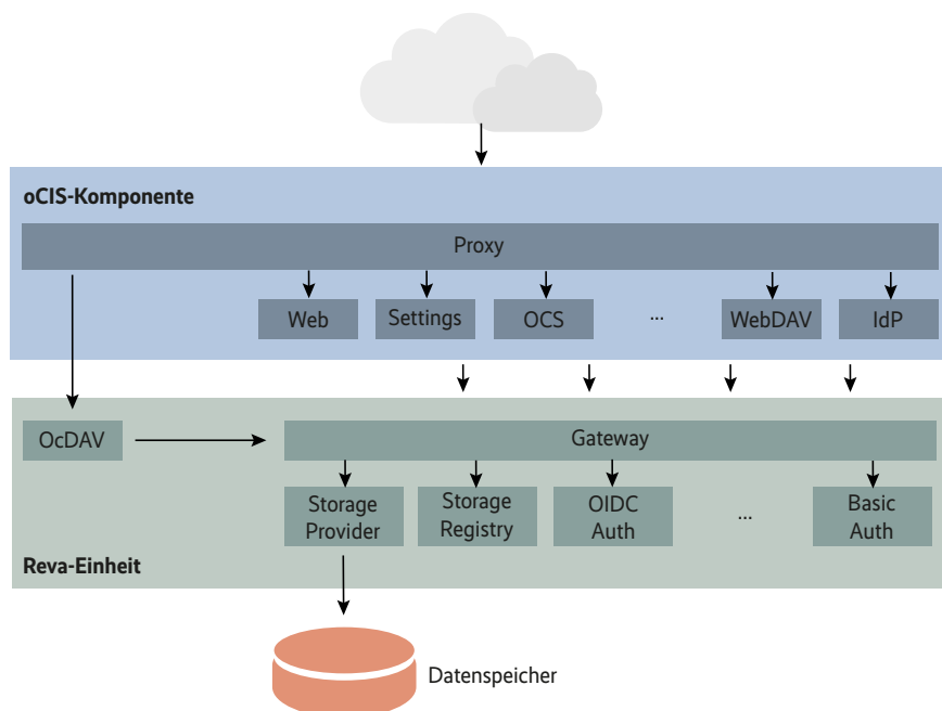
Für oCIS setzt ownCloud auf eine dreischichtige Microservice-Architektur (Abb. 1).
